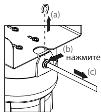
Отсоединение трубок
