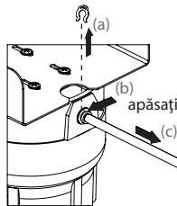
Scoaterea tubului
